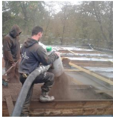
5 - Soufflage sur la toiture du substrat JARDILIGHT 1.1 POTAGER pour les potagers urbains. ECOVEGETAL a sa propre flotte de camions silos.
